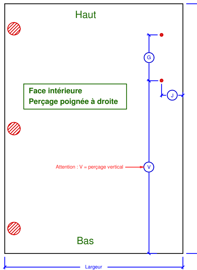
Poignée verticale
