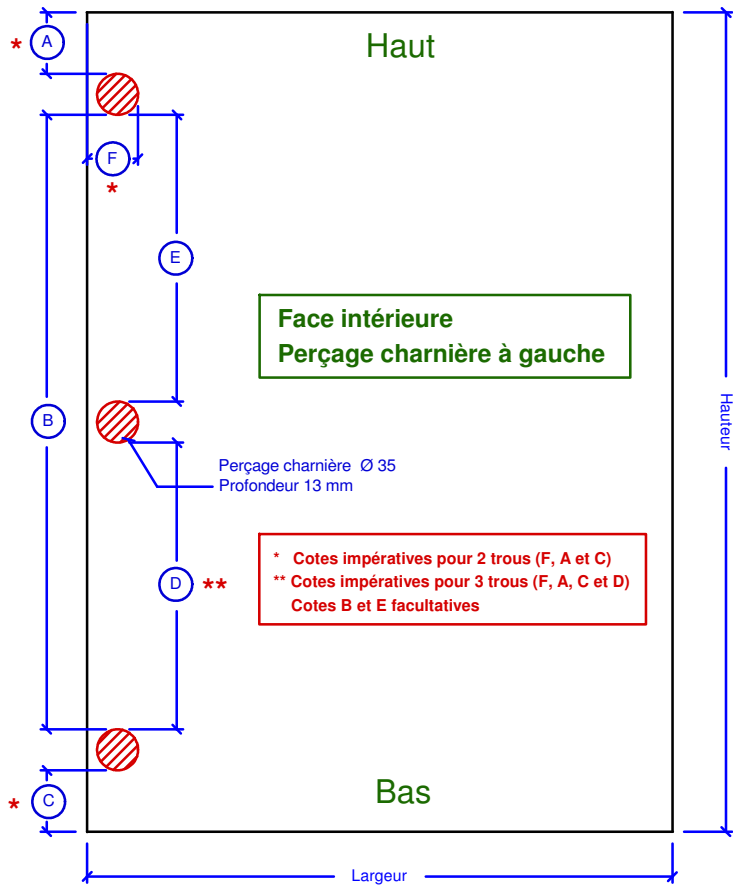
Charnière
